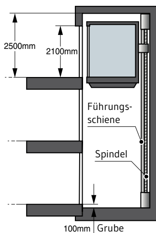
Spindelgetriebener Lift
