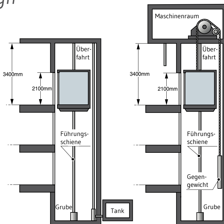
Hydraulikaufzug
